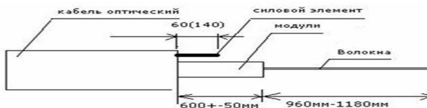
Рисунок 2. Разделка кабеля
