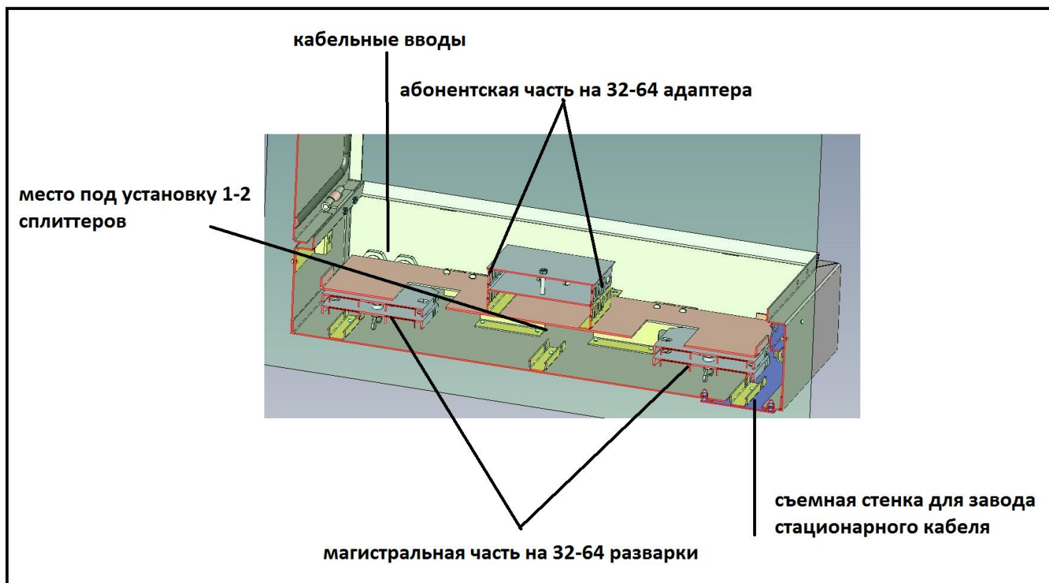
Схема расположения оборудования
