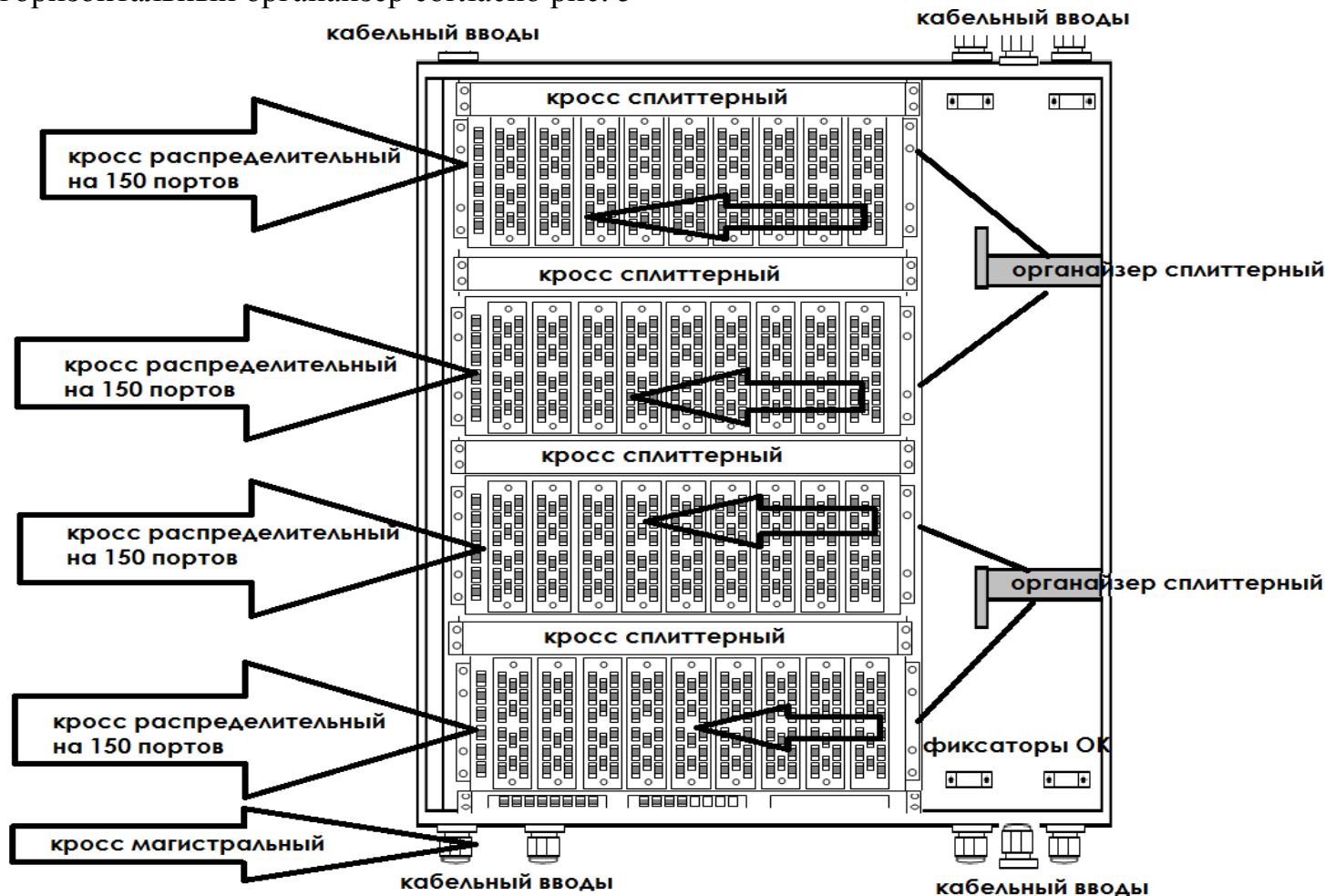
Рис. 5 Кабельные магистрали
