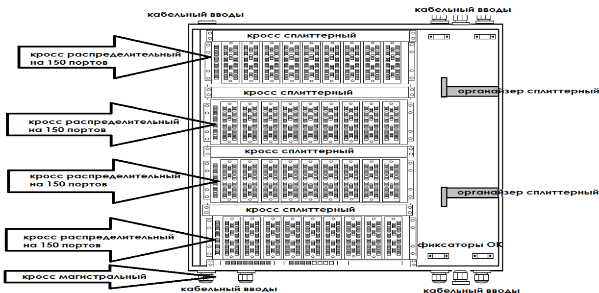
Схема расположения оборудования
