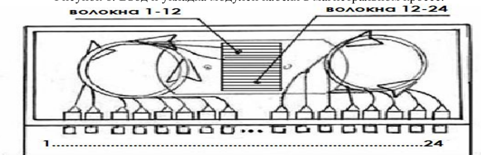
Рисунок 6. Схема укладки пигтейлов.
